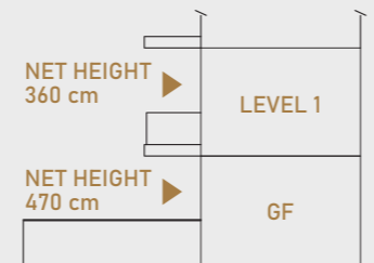
DUPLIX ELEVATION
